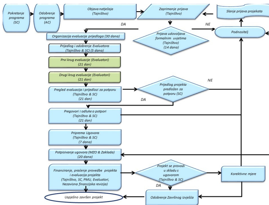
Slika 2b: Dijagram toka od prijave do završenog projekta u slučaju dva kruga evaluacije
